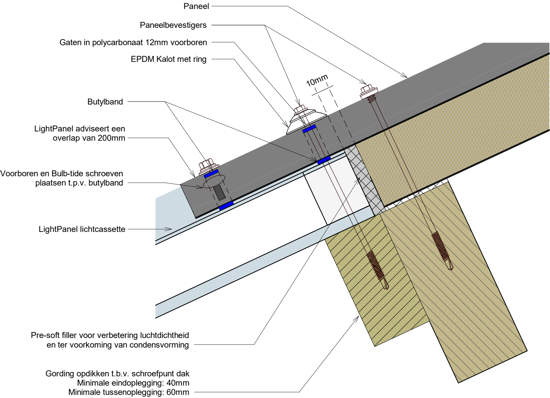
1 Detail-boven 1 : 2
